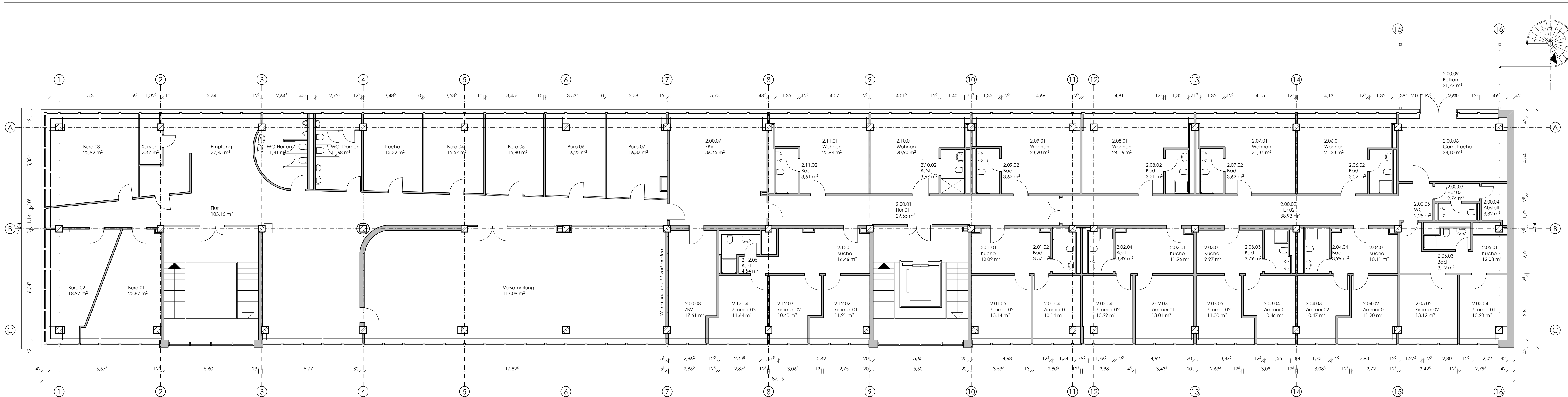
Grundriss 2.OG
